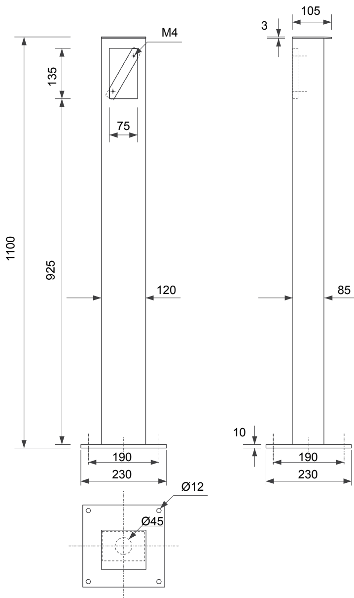
Maßskizze GSB Säule für PKW (Maße in mm)
