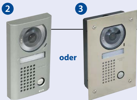
JF-DV (Aufputz, Zinkdruckguss) 173 x 98 x 27mm EL-12S Türöffner oder pot.freier Schließer (ohne Trafo) JF-DVF (Unterputz, Edelstahl) 209 x 135 x 5,5 / 45mm
